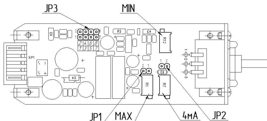
Рисунок 2- Расположение блоков переключателей и органов регулировки выходного сигнала внутри блока ручного управления БПУ-1
